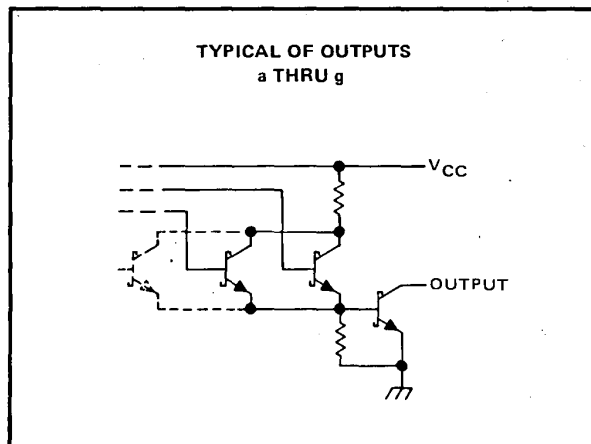
'LS249
