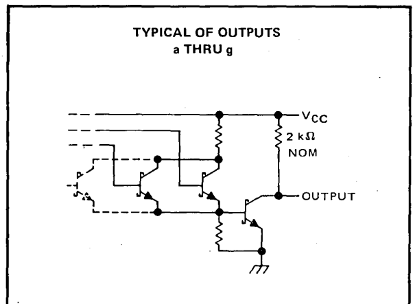
'LS248
