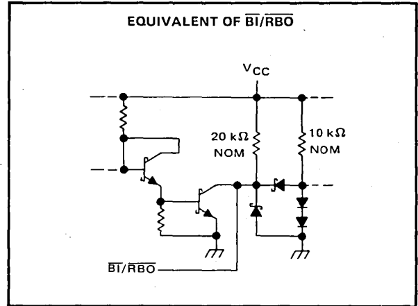
'LS248
