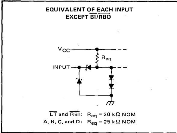
'LS247
