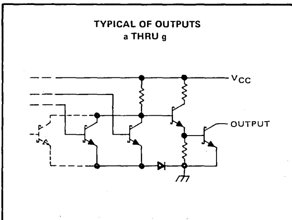
'LS247
